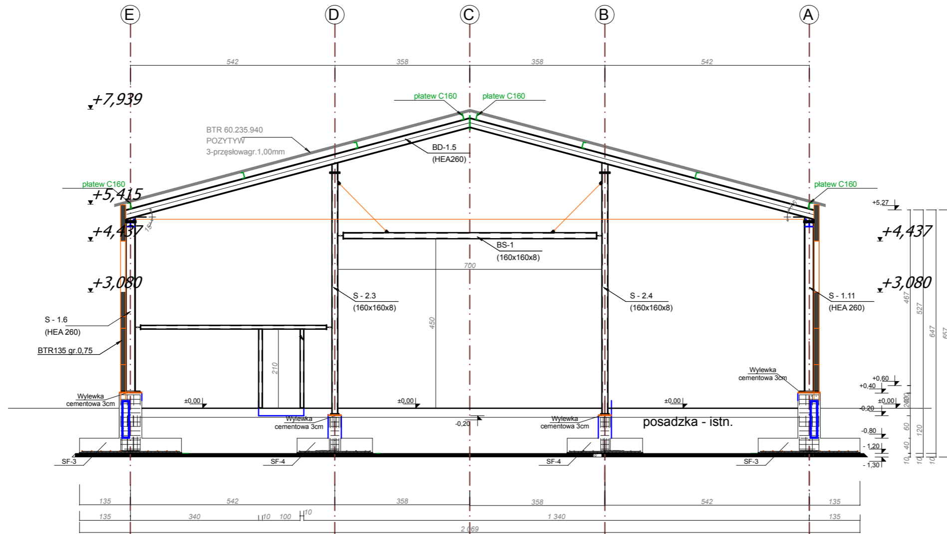
przekrój a-a
